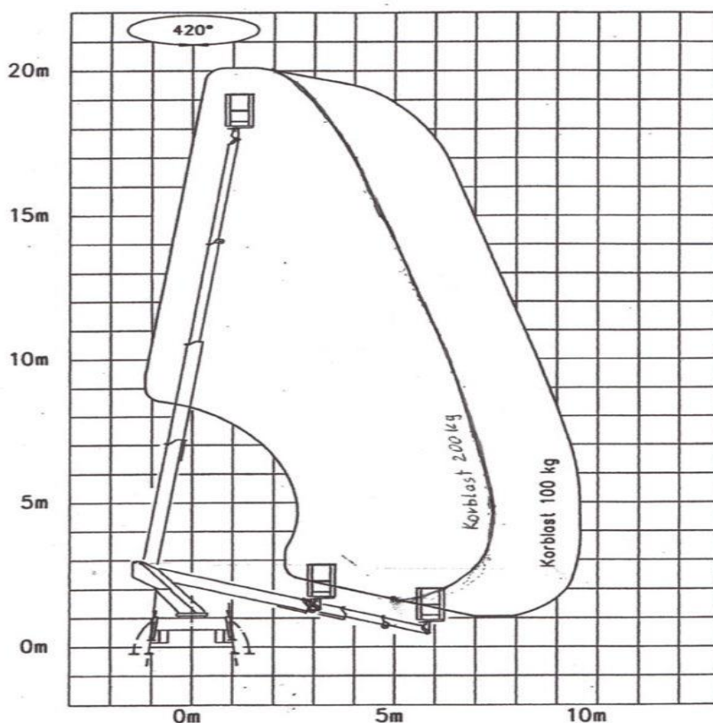
Arbeitsdiagramm WT200 WUMAG elevant
